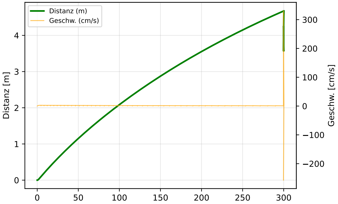
Fahrzeugbewegung
