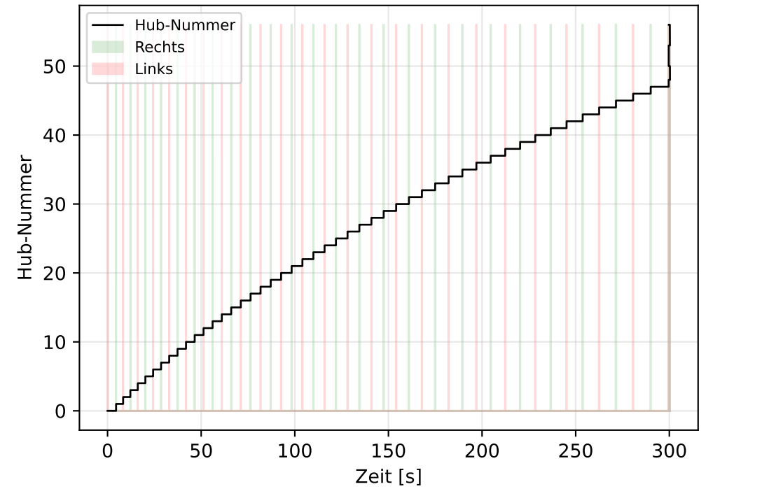
Kolben-Hübe
